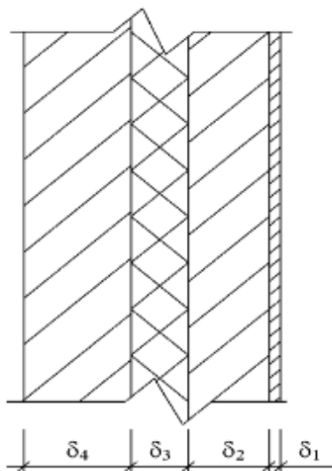
Рисунок – Трехслойная наружная стена
